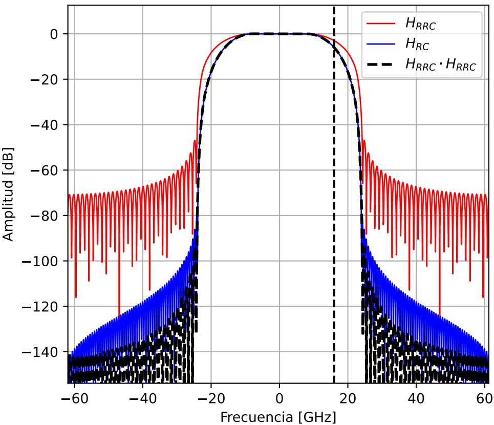
Respuesta en Frecuencia del RC y RRC. \beta = 0.5
